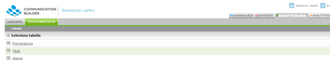
Figura 57 - Configurazione tabelle
