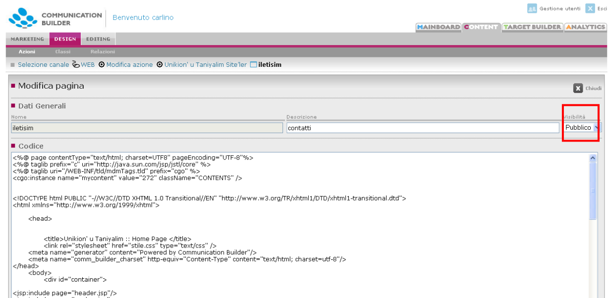
Figura 35 – Una scena
